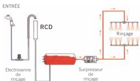
Cycle de rinçage avec système RCD
